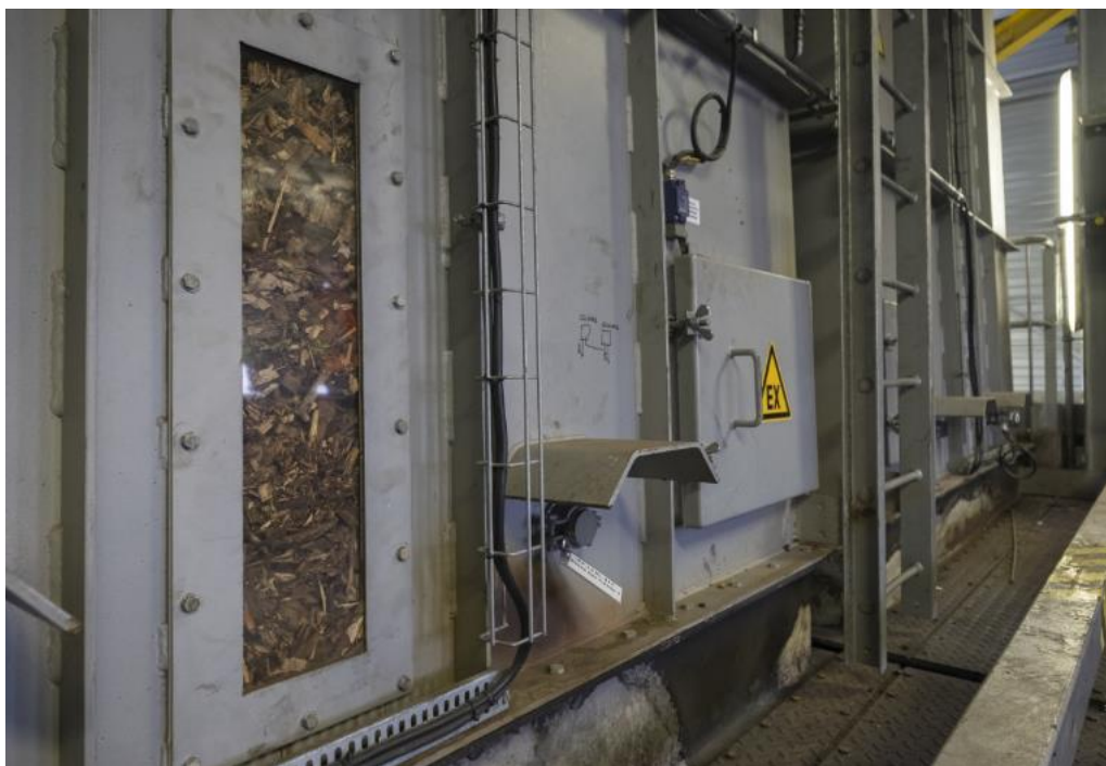
Arrivée des plaquettes dans une chaudière à bois
