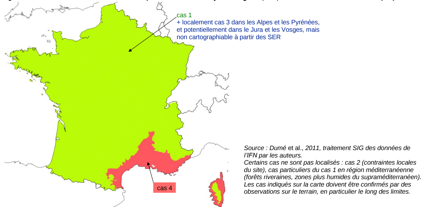
Figure 2 – Localisation indicative des cas IBP à partir de la carte des sylvoécotérrains (SER) de l'Inventaire Forestier National (IFN)
